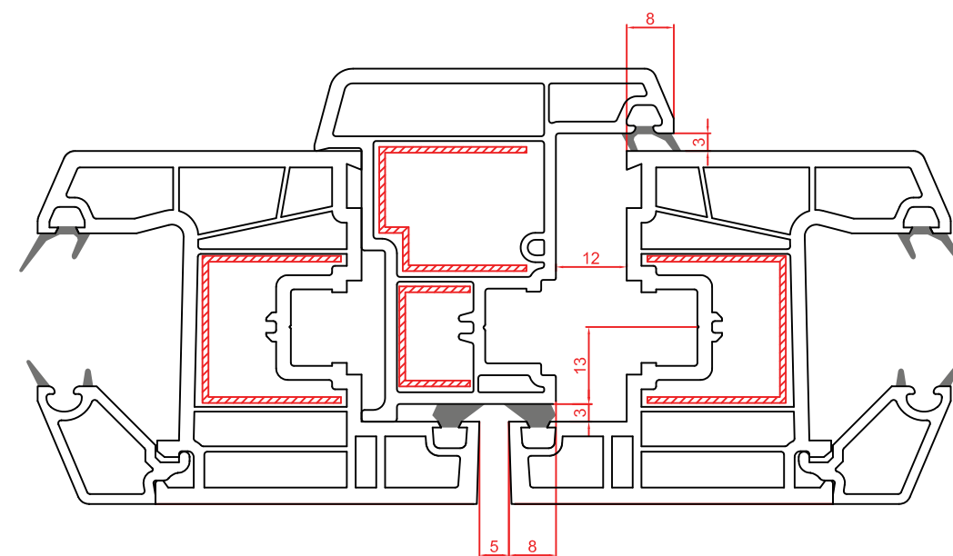
Moveable Mullion Assemble Figure التجمع المنقولة
